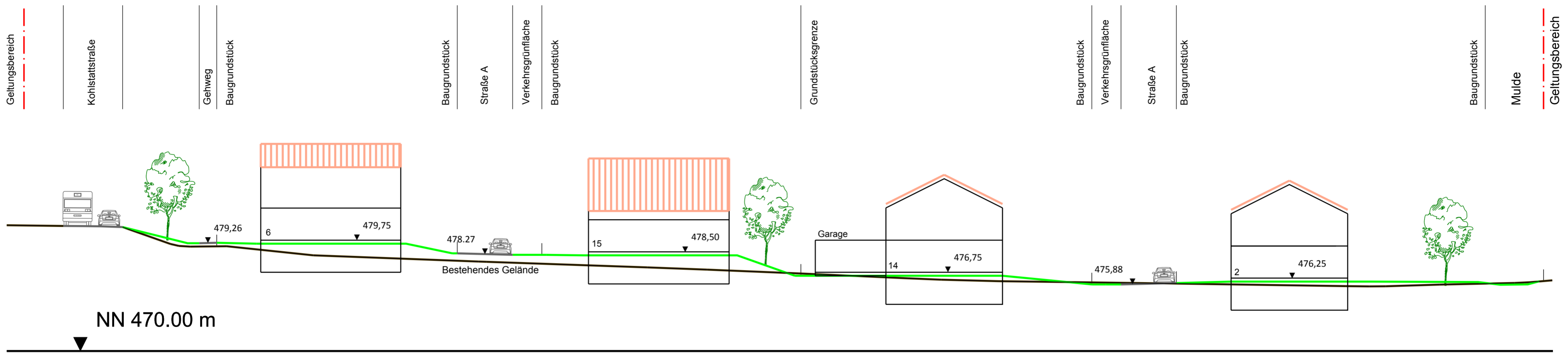
Schnitt 1 - 1
