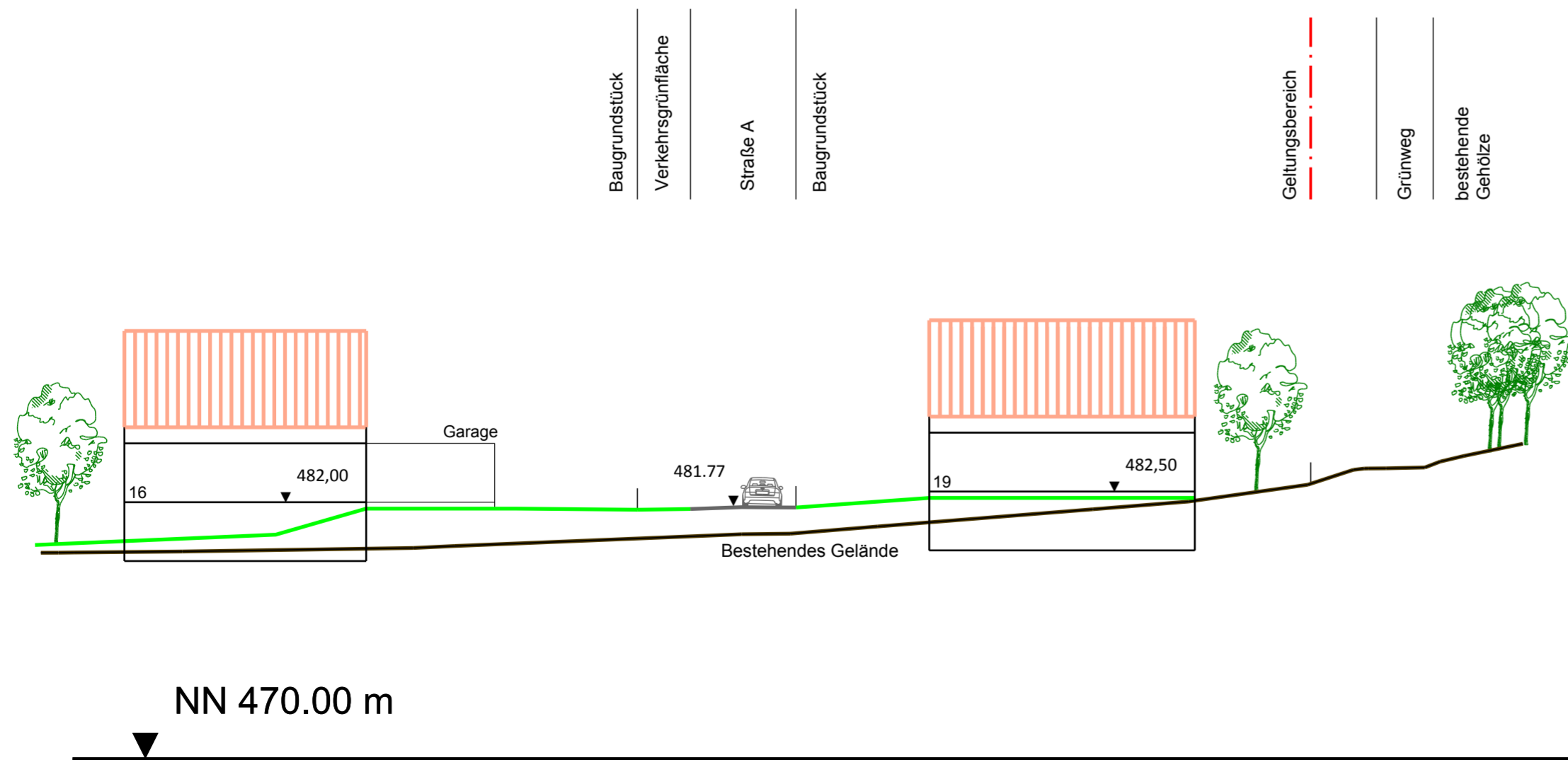
Schnitt 3 - 3
