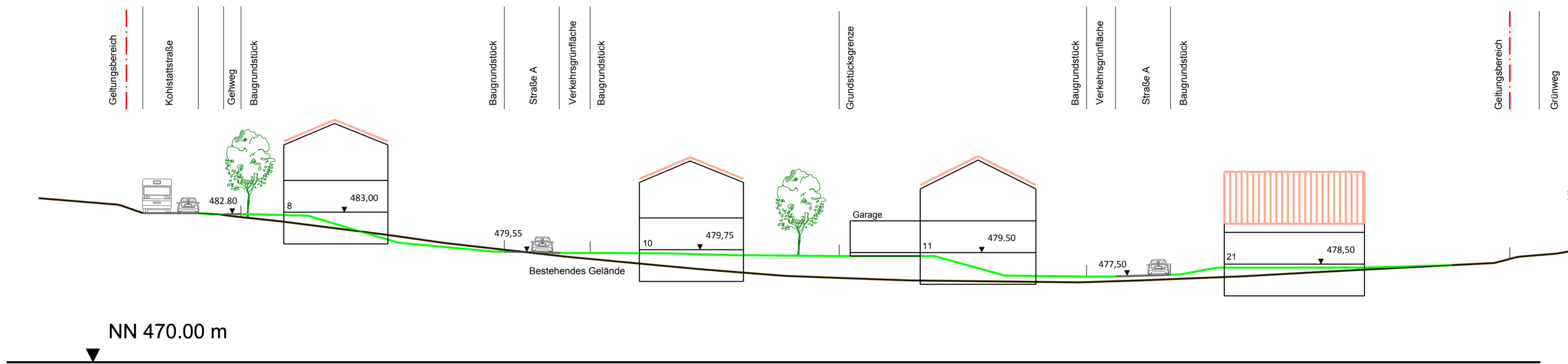
Schnitt 2 - 2
